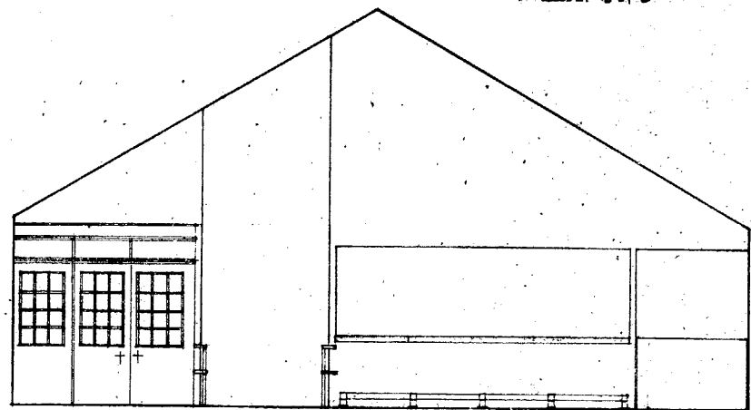
ELEVATION 13
