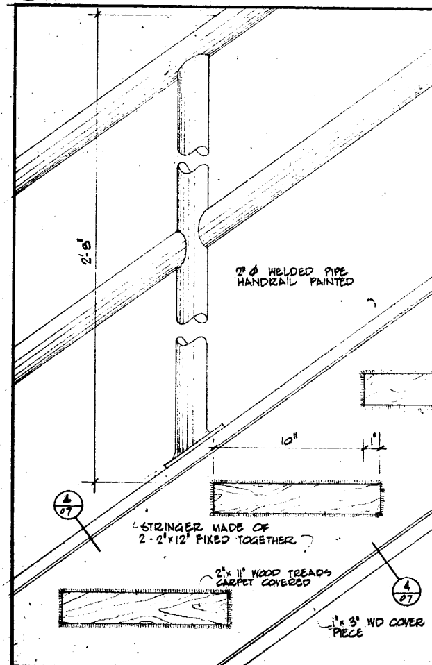
SECTION THRO BAR SCALE: 1/4" = 1'-0"
