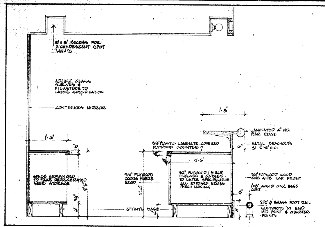
SECTION THRO BAR SCALE: 1/4" = 1'-0"
